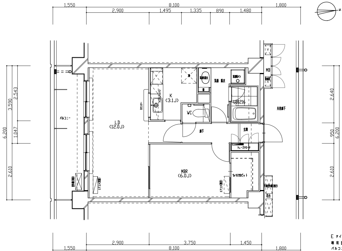
Eタイプ平面図 S=1/100
